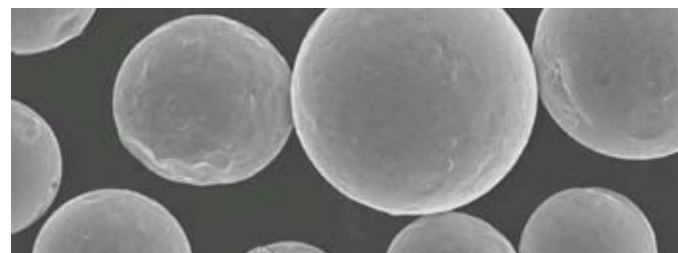
Figura 8 Partículas esféricas de pós de base Ni sem presença de satélites
