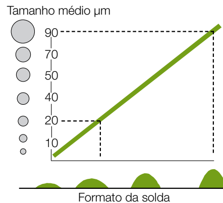
Figura 13 Efeito do tamanho de partícula no formato do cordão de solda
