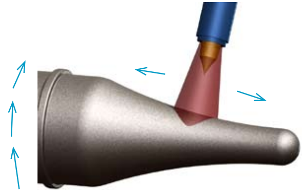
Figura 23 Fusão dos punções
