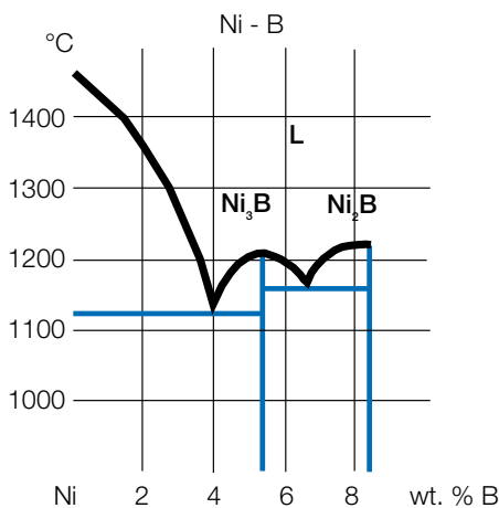
Figura 2a Diagrama de fases para o Ni-B
