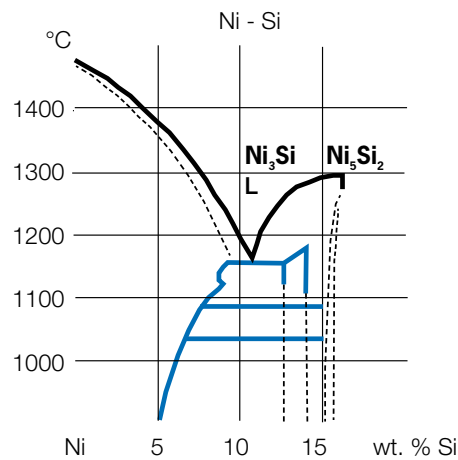
Figura 2b Diagrama de fases para o Ni-Si
