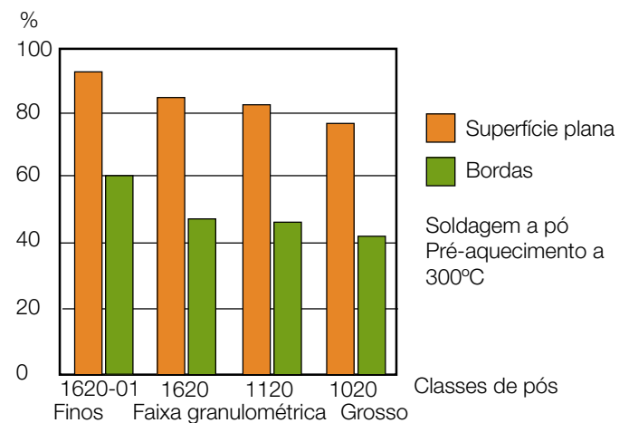
Figura 14 eficiência da deposição
