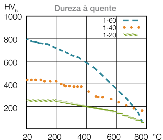
Figura 6 O efeito da temperatura na dureza
