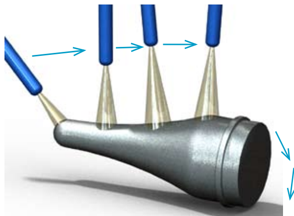
Figura 22 Inicie a aspersão pelo topo dos punções
