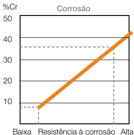
Figura 5 Ni, Cr, Mo and Cu aumentam a resistência à corrosão, C e B reduzem.
