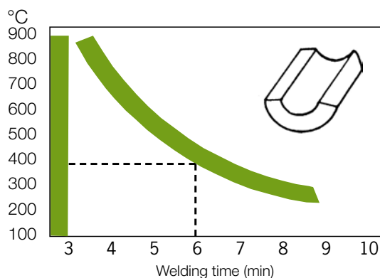
Figura 17 Importância do pré-aquecimento no tempo de solda
