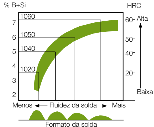
Figura 12 Efeito do B + Si na fluidez e dureza
